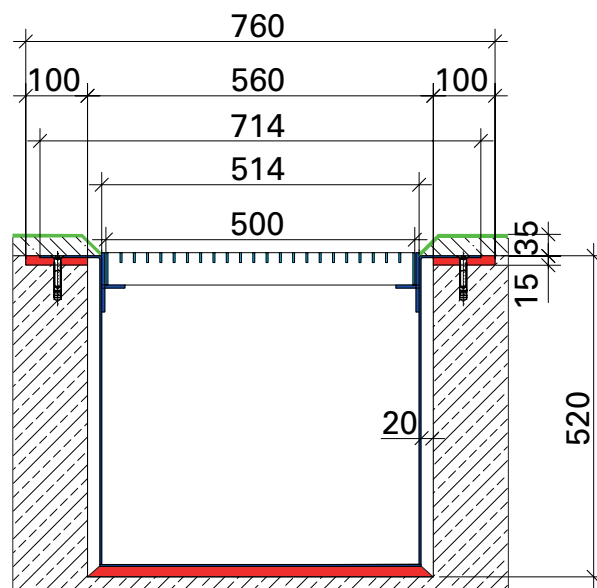
Querschnitt Mulde
