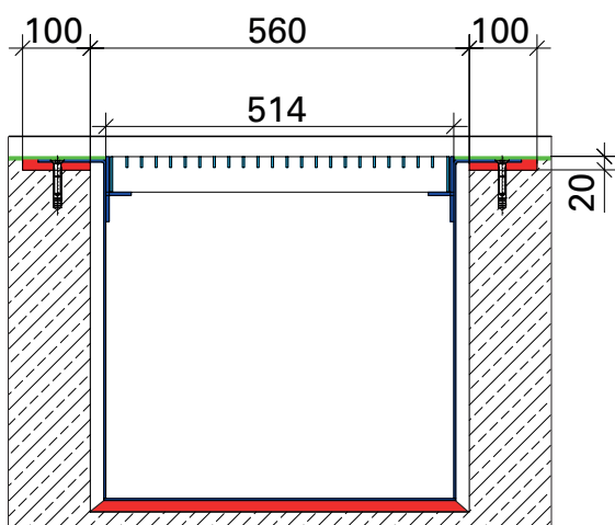
Längsschnitt
